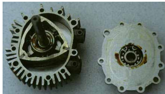
Moteur rotatif
