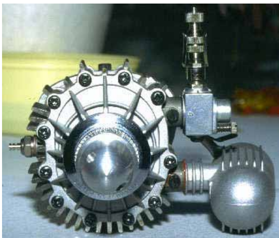
Moteur rotatif
